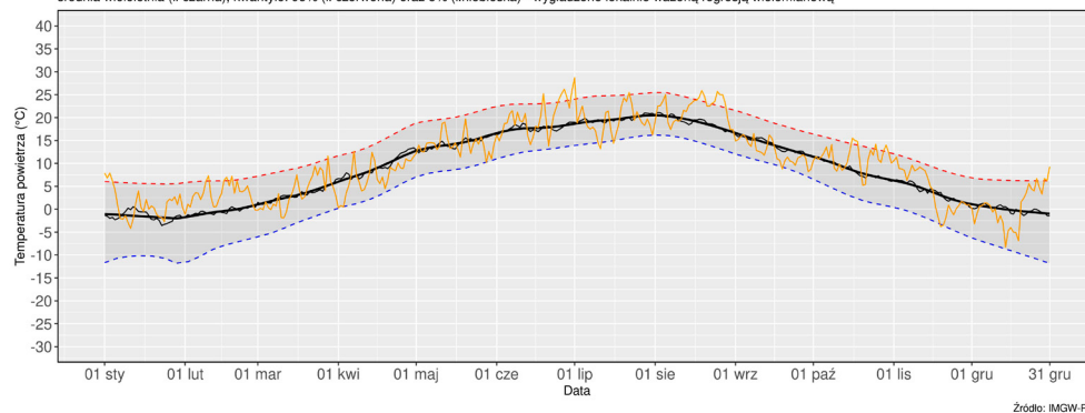
KROSNO - zmienność średniej dobowej temperatury powietrza (TSRD) w 2022 na tle charakterystyk wieloletnich 1991-2020 średnia dobowa 2022 (l. pomarańczowa), średnia wieloletnia (l. czarna), kwantyle: 95% (l. czerwona) oraz 5% (l. niebieska) - wygładzone lokalnie ważoną regresją wielomianową
