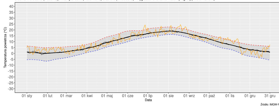
WARSZAWA_OKĘCIE - zmienność średniej dobowej temperatury powietrza (TSRD) w 2022 na tle charakterystyk wieloletnich 1991-2020 średnia dobowa 2022 (l. pomarańczowa), średnia wieloletnia (l. czarna), kwantyle: 95% (l. czerwona) oraz 5% (l. niebieska) - wygładzone lokalnie ważoną regresją wielomianową
