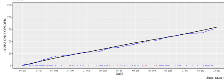
Skumulowana liczba dni z opadem (dobowa suma opadu \geq 0.1\text{mm} ) w roku 2022 - I. niebieska na tle skumulowanych średnich miesięcznych liczby dni z opadem w wieloleciu 1991-2020 - I. czarna pogrubiona, punkty niebieskie - dni z opadem, czerwone - dni z opadem > 10\text{mm} WŁODAWA
