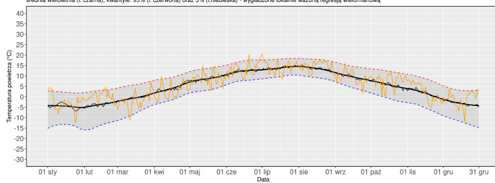
KROSNO - zmienność minimalnej dobowej temperatury powietrza (TMIN) w 2022 na tle charakterystyk wieloletnich 1991-2020 minimalna dobowo temperatura powietrza w 2022 (l. pomarańczowa), średnia wieloletnia (l. czarna), kwantyle: 95% (l. czerwona) oraz 5% (l. niebieska) - wygładzone lokalnie ważoną regresją wielomianową
